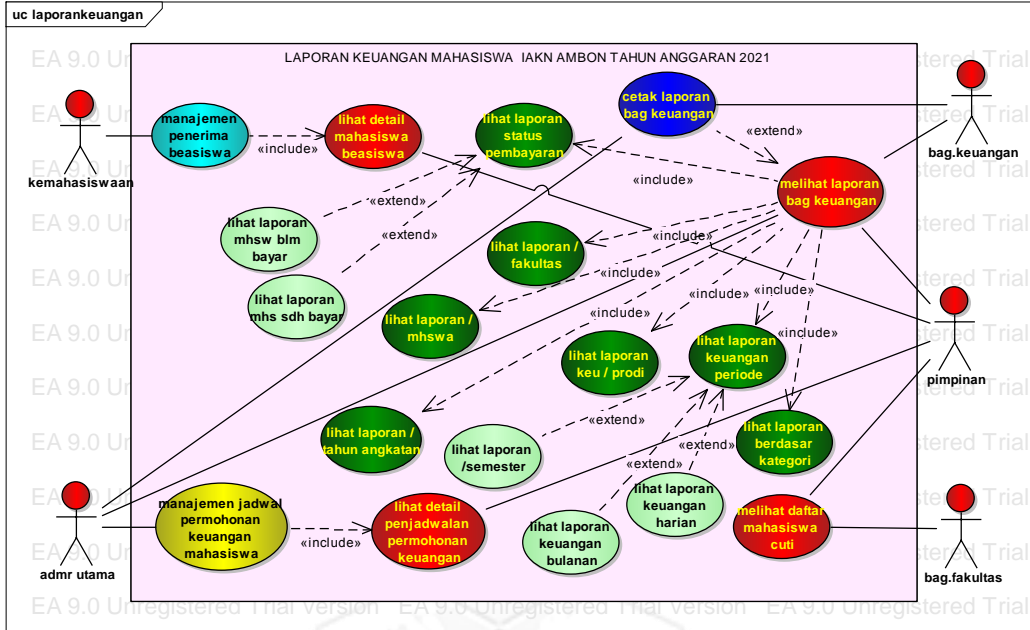
Gambar 2. Use Case Keuangan Mahasiswa IAKN Ambon (level 2)
